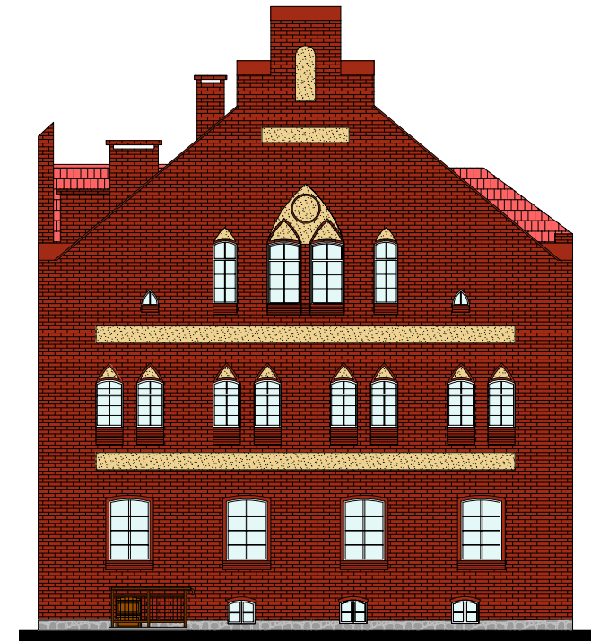
ELEWACJA POŁUDNIOWA
