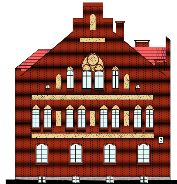
ELEWACJA PÓŁNOCNA
